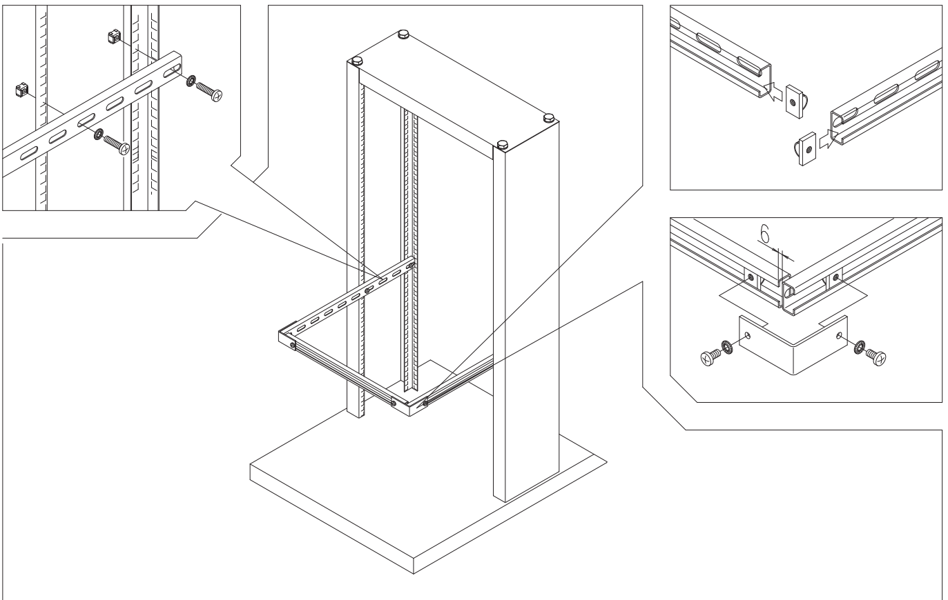
Kabelabfangschiene
