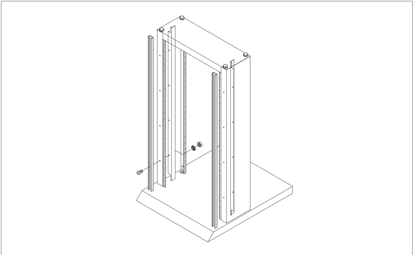
Montageprofil 19"-Rasterprofil
